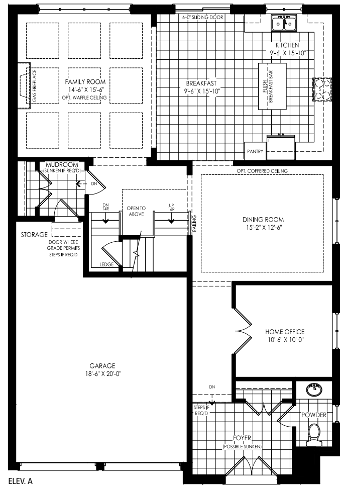
ELEV. A
