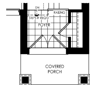
ELEV. B
