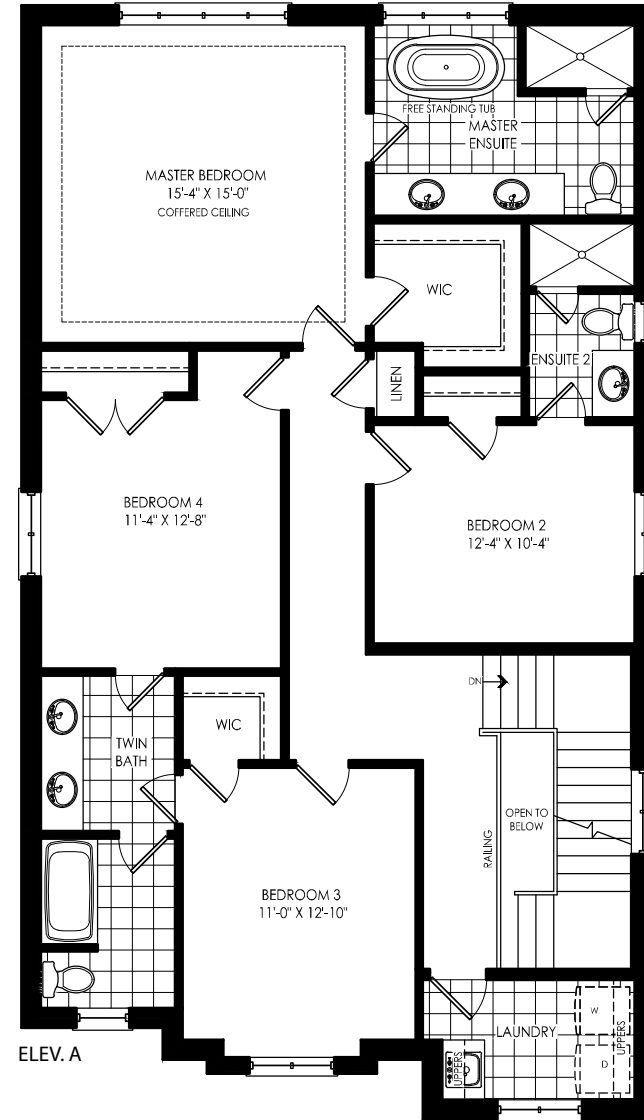
ELEV. A
