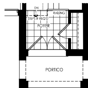
ELEV. C
