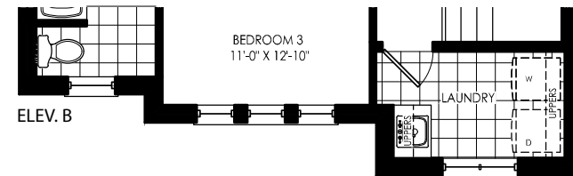
ELEV. B
